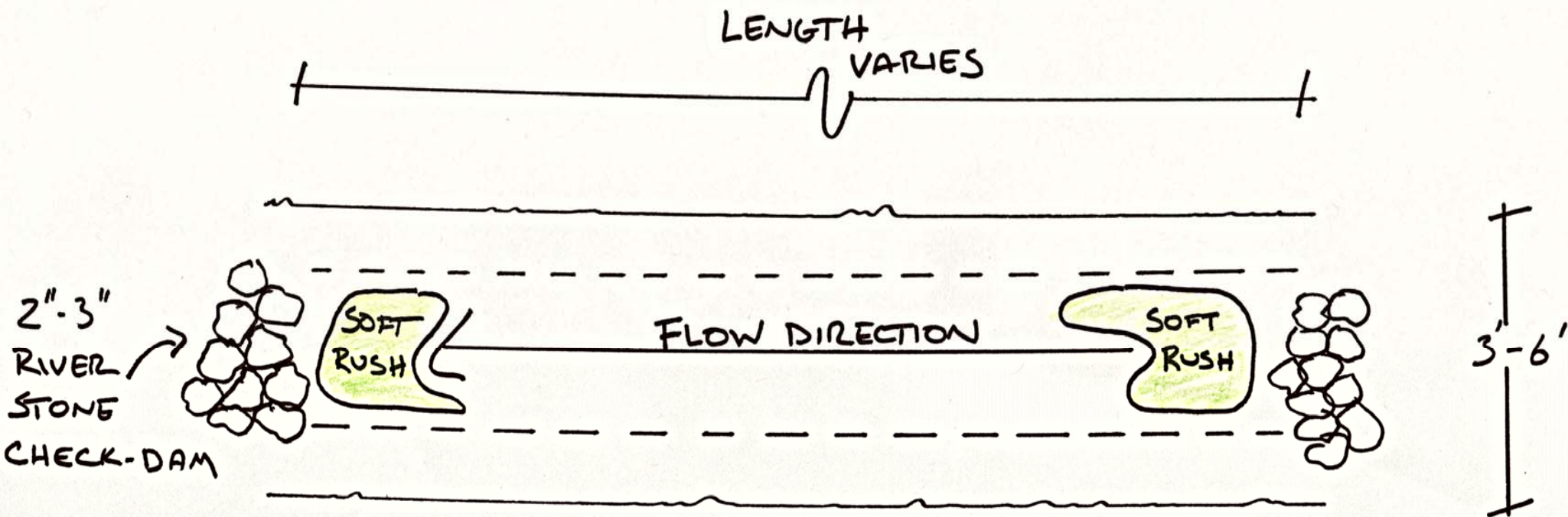
BIOSWALE - PLAN
